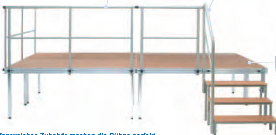
Bühne mit geeignetem Belag auch im Außenbereich verwendbar
