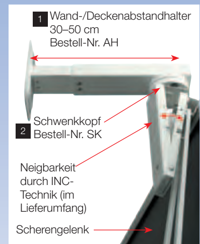
Rückansicht mit Abstandhalter und Schwenkkopf, geneigt
