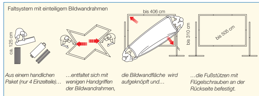
Automatisch einrastende, stabile Schnappgelenke an Rahmen und Fußstützen
