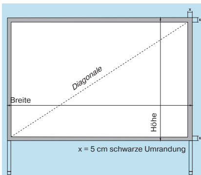
Bildwandfolie mit 5 cm breiter schwarzer Randverstärkung
