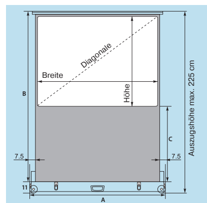
Rollen und Handgriff für einfachen Transport
