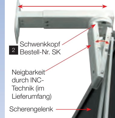
Rückansicht mit Abstandhalter und Schwenkkopf, geneigt
